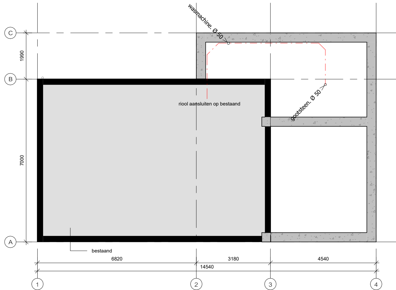
fundering/palenplan paaltype: stalenbuispalen conform opgave constructeur funderingsbalk: conform opgave constructeur
