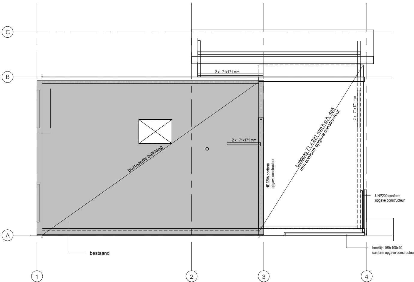
1e verdiegingsvloer
