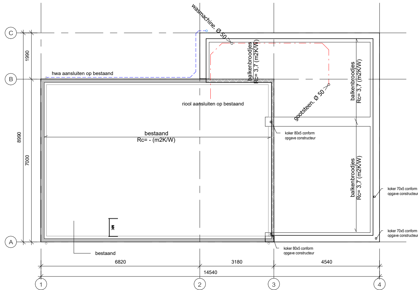
vloerenplan begane grond - PS-combinatievloer conform opgave constructeur
