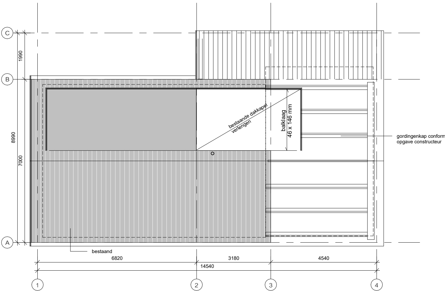
dakconstructie gordingkap: conform opgave constructeur
